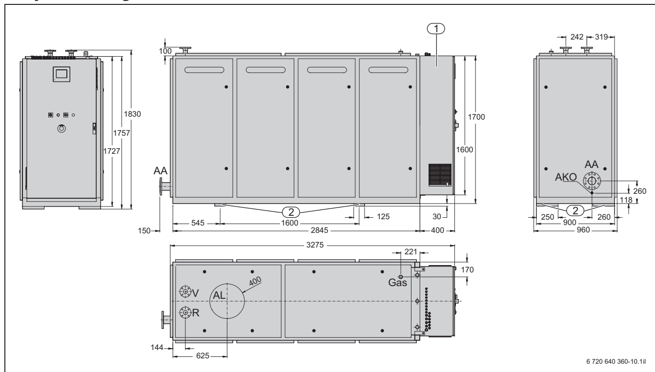
Рис. 13. Размеры и подключения модуля ВНКW Loganova EN70 (Размеры в мм, подключения см. табл. 12)
