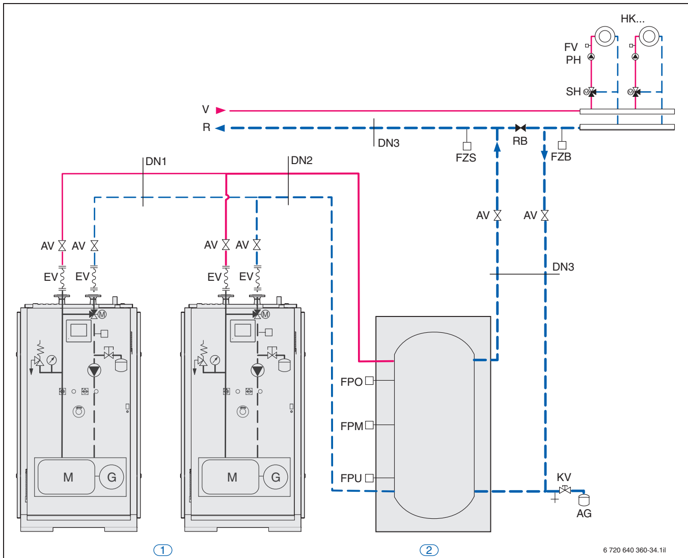
Рис. 43. Гидравлическая схема двух модулей ВНКW Loganova с буферным тепловым аккумулятором и регулированием с помощью буферного бака-аккумулятора типа Premium
