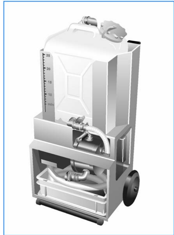
96/1 Заправочная станция Logasol BS01.
