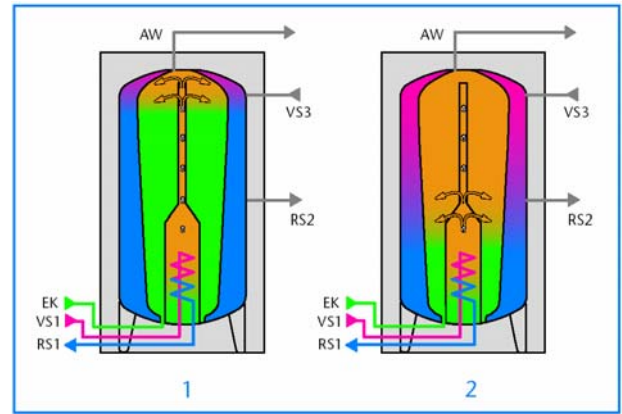
18/1 Заполнение термосифонного комбинированного бойлера с помощью теплообменника гелиоконтра (1) и замедленное заполнение буферного аккумулятора горячей воды (2).
