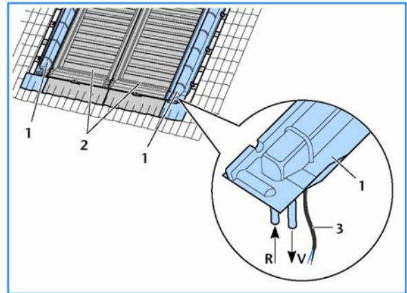
105/1 Гидравлическое подключение под крышей в случае монтажа в крышу с применением поддонов. Существует возможность установки дополнительного развоздушителя в верхней зоне боковины гелиоколлекторного поля (над крышей).
