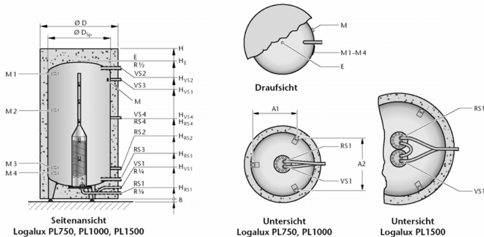
22/1 Габаритные размеры и места присоединения (подключения) термосифонных буферных бойлеров Logalux PL...
