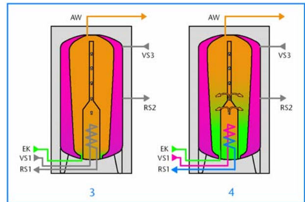
18/2 Отбор горячей воды из полностью заполненного бойлера (3) и пополнение холодного снизу накопителя расходной воды с помощью теплообменника гелиоконтра, хотя буферный аккумулятор горячей воды ещё полный (4).
