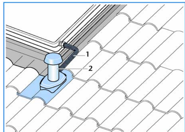
107/3 Кровельный проход для присоединительного обратного трубопровода комплексной гелиостанции KS... с подъёмным уклоном к развоздушивателям.
