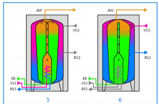
18/3 Пополнение накопителя расходной воды с помощью теплообменника гелиоконтра и буферного аккумулятора горячей воды (5), а также дополнительный нагрев от обычного (традиционного) котла отопления в случае недостаточного гелиотермического выхода (6).
