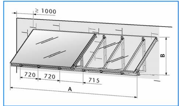
77/2 Монтажные размеры фасадных комплектов с фиксированным углом наклона 45° для плоских гелиоколлекторов Logasol SKN2.0-w и SKS3.0-w горизонтального типа (Размеры A и B в мм смотри 77/1).
