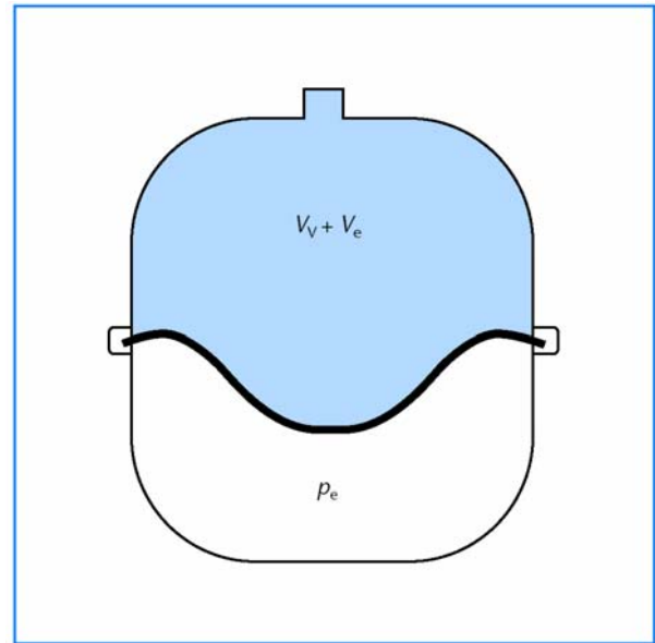
91/2 Остаточное давление мембранного компенсационного бака.
