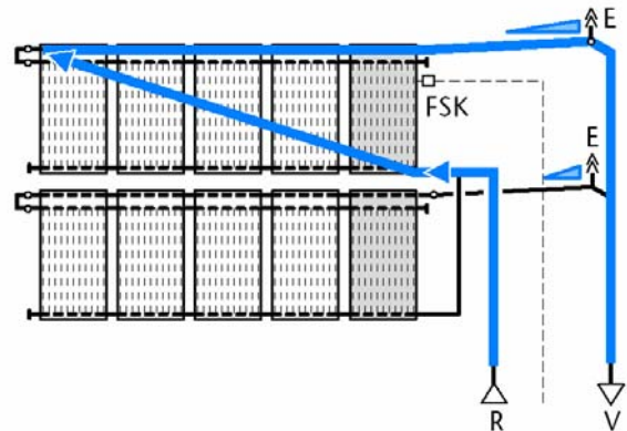
84/3 Параллельное соединение двух рядов гелиоколлекторов Logasol SKS3.0 по принципу Тихельманна.
