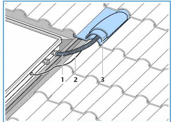
107/2 Кровельный проход присоединительного прямого трубопровода с подъёмным уклоном к развоздушивателю в случае применения комплексной гелиостанции KS...
